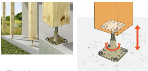
Fijación pie de pilar PPRC sobre soporte rígido
